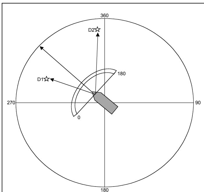
Figuur 2.10. Overzicht van de verschillende hoeken die gemeten zijn voor 2 duikers (D1 en D2). De vaarrichting bedraagt 315°. De hoek van waarnemen bedraagt 290° voor duiker D1 en 5° voor duiker D2. De hoek van waarnemen ten opzichte van de vaarrichting bedraagt 65° voor duiker D1 en 140° voor duiker D2.
