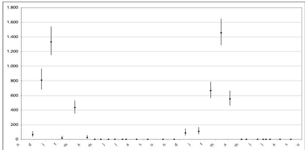
Figuur 4.3. Totaal aantallen van roodkeelduiker op open water (en de kustzone) van de Voordelta op basis van geëxtrapoleerde transecttellingen per vliegtuig op grond van de stripbandmethode (alleen vogels in AB-strip). Weergegeven zijn 95% betrouwbaarheidsintervallen op basis van een GLM-analyse (factoren telling en deelgebied).
