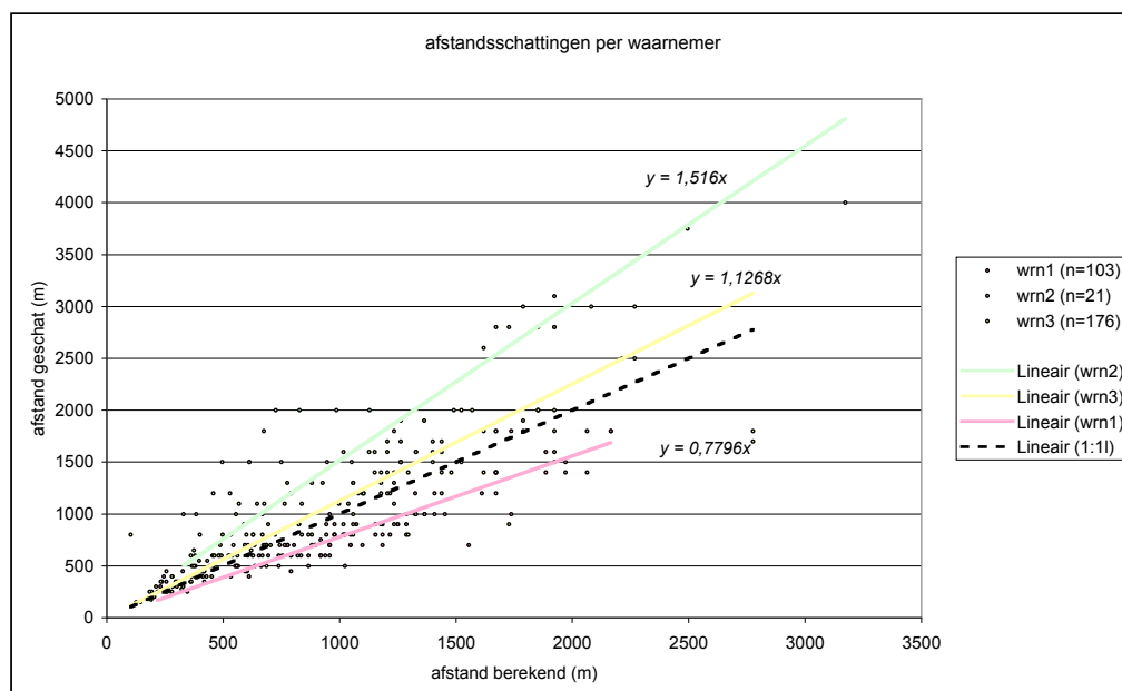
Figuur 2.11. Geschatte afstand tot waargenomen duikers vergeleken met berekende afstand tot duikers. Berekende afstanden zijn m.b.v. de schuifmaat bepaald. Voor iedere waarnemer is een lineaire trendlijn door de oorsprong berekend.
