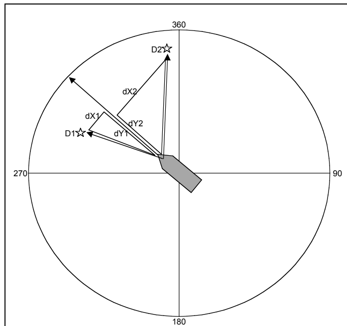
Figuur 2.12. Relatieve afstand van 2 duikers (D1 en D2) ten opzichte van de boot in de X-richting ( dX ) en Y-richting ( dY ) berekend op basis van de hoek van waarnemen en de absolute afstand van de betreffende duiker tot de boot.
