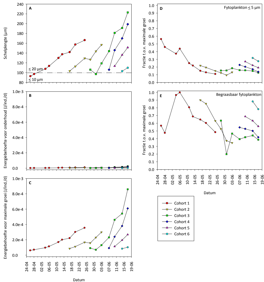
Figuur 17 Input (links) en resultaten (rechts) van de modellering van de energieopname van schelpdierlarven in de Haringvlietmonding, april tot en met juni 2010. A) lengte van de veligers in de verschillende cohorten (zie legenda) aan de hand van de frequentieverdelingen uit Figuur 14. B) energiebehoefte voor onderhoud (= minimale energiebehoefte) van de schelpdierlarven. C) energiebehoefte voor maximale groei. D) verhouding tussen de gemodelleerde groei en de maximale groei bij opname van alleen klein fytoplankton ( \leq 5 \mu\text{m} , bovenste figuur) of E) opname van de begraasbare grootteklassen van het fytoplankton (alle deeltjes \leq 10 \mu\text{m} of \leq 20 \mu\text{m} , afhankelijk van schelpenlengte). In figuur A is aangegeven welke fractie van het fytoplankton naar verwachting door de schelpdierlarven begraasd kan worden: larven kleiner dan 50 \mu\text{m} kunnen zich alleen voeden met fytoplankton \leq 5 \mu\text{m} , larven groter dan 100 \mu\text{m} begrazen de eerste drie grootteklassen van het fytoplankton (alle deeltjes kleiner dan 21 \mu\text{m} ). Tussen een schelpenlengte van 50 en 100 \mu\text{m} begrazen larven alleen de eerste twee fracties (tot en met 10 \mu\text{m} ). Gegevens gebaseerd op de gemiddelde voedselbeschikbaarheid van LOCATIE 1, 2 en 3.
