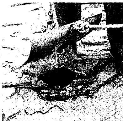
Fig. 2.1. Monstertuigen die worden gebruikt bij de kokkelinventarisatie (links het kokkelschepje, rechts de stempelkor).
